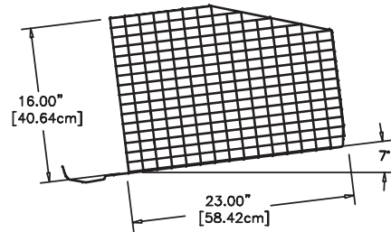
Partición o División de Jaula (Piso Superior)
